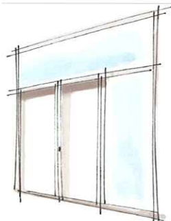
DOPPIO BATTENTE CON SOPRALUCE E SINGOLO FIANCOLUCE
