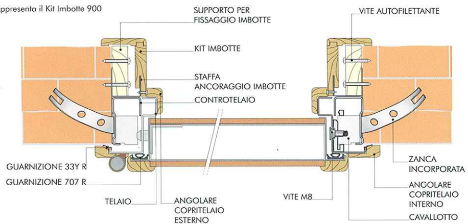
MONTAGGIO CON FINITURA LEGNO
