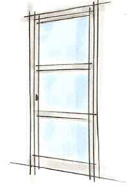
PORTA FINESTRA A UN BATTENTE CON DUE TRAVERSINE
